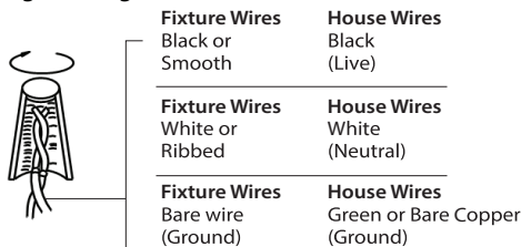
Fig. 2 Wiring
