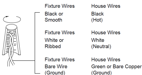
Fig. 2 Wiring
