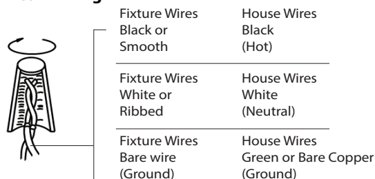
FIG. 2 Wiring
