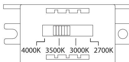
Fig. 3 Switch
